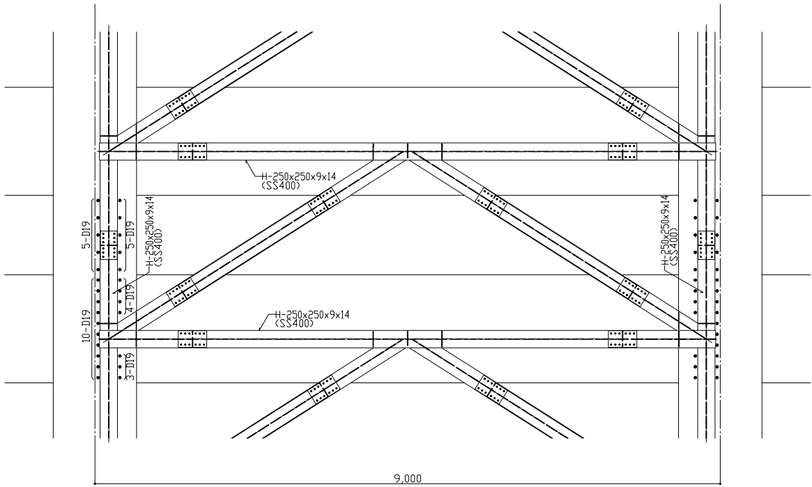
ブレース K1型 1/30
