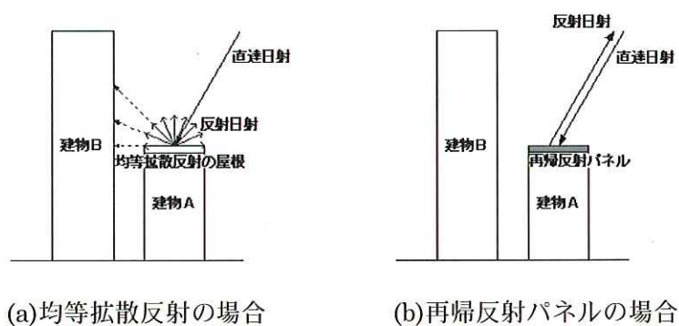
図 1 再帰反射パネルの設置例
