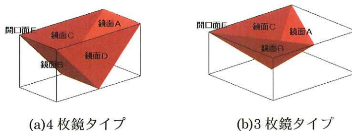
図 2 再帰反射ユニットの形状
